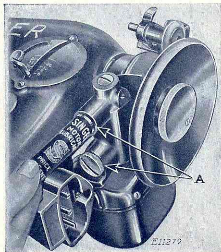
FIG. 29. LUBRICATING THE MOTOR
